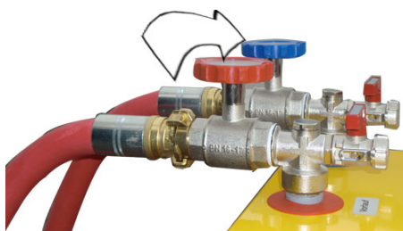
Bild: Kugelhähne mit Thermometergriff schließen
